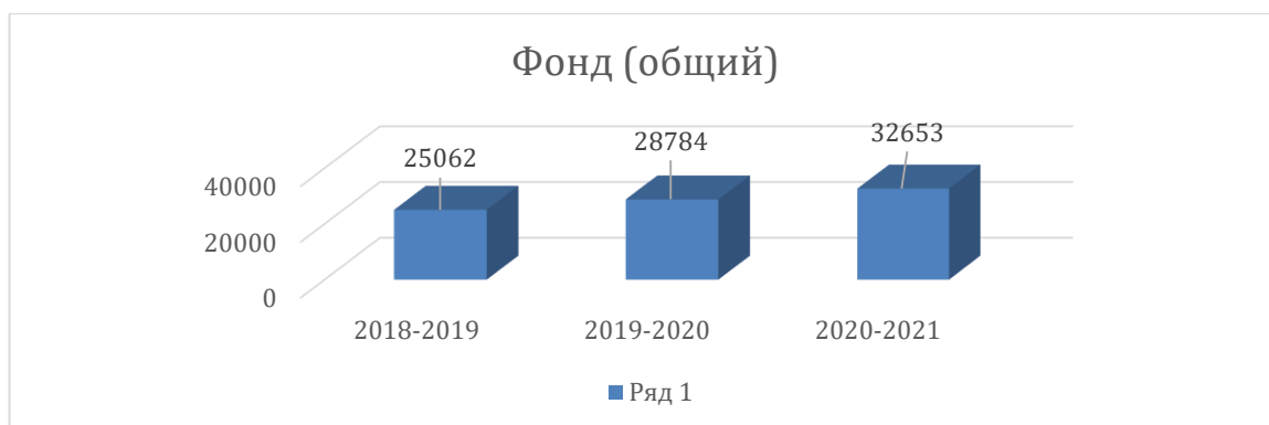
Диаграмма 3
